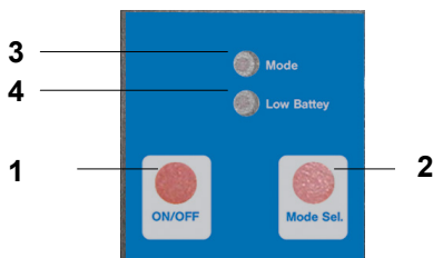
Figure 2 : Éléments de commande Wöhler US 23 Émetteur
